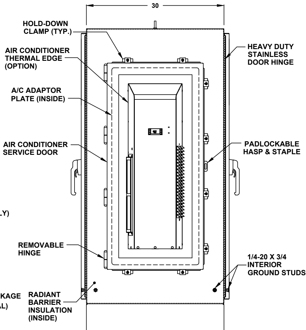
LEFT SIDE
