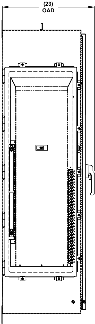
LEFT SIDE
