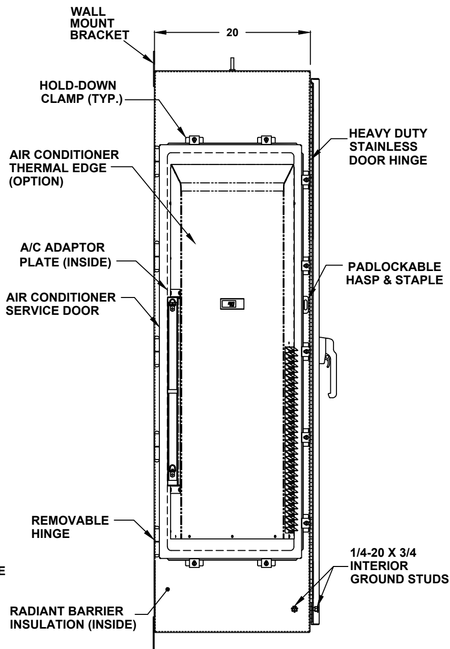
LEFT SIDE
